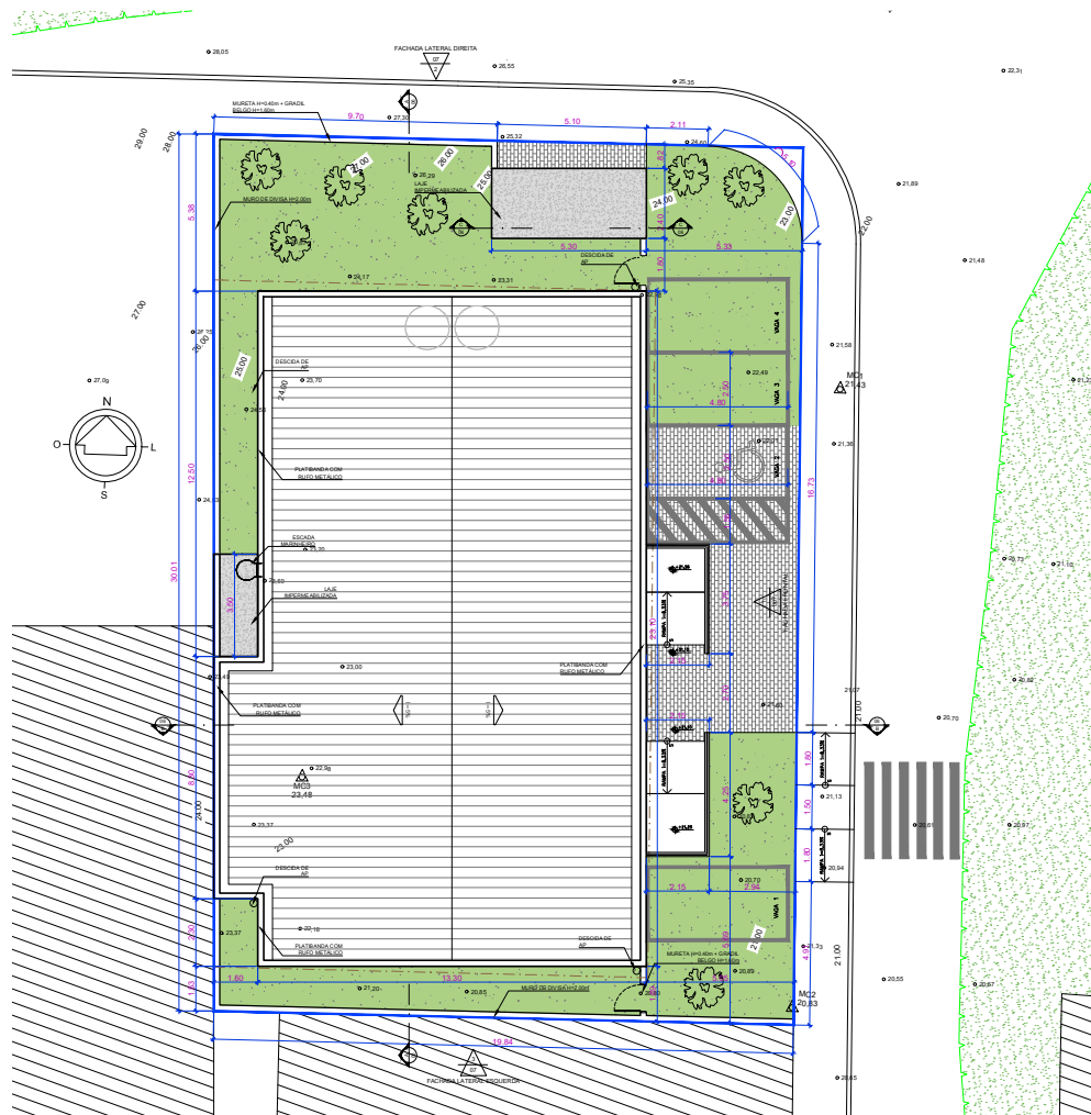
1 IMPLANTAÇÃO COM COBERTURA ESCALA 1/100
