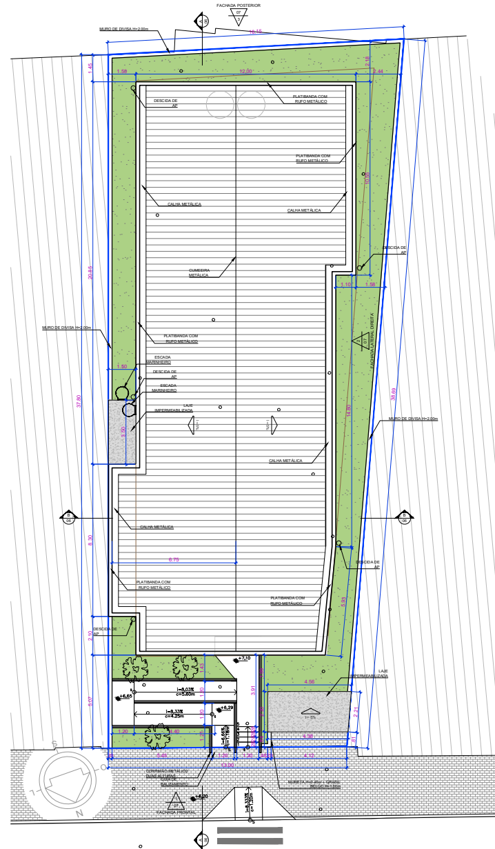
1 IMPLANTAÇÃO COM COBERTURA ESCALA 1/100
